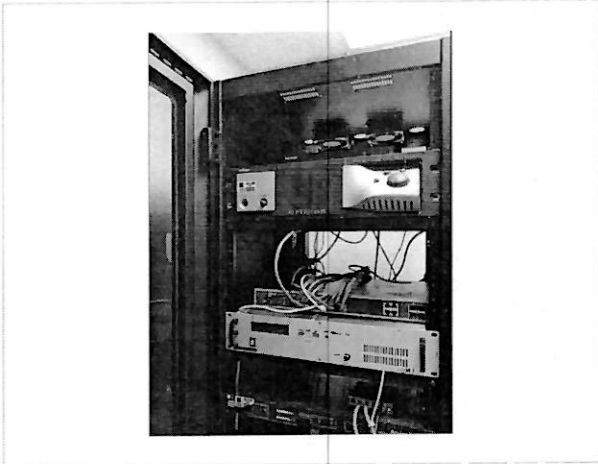
Se coloca el procesador de audio en el rack de equipos, se enciende y se conectan los cables de poder, de entrada y salida de audio.
