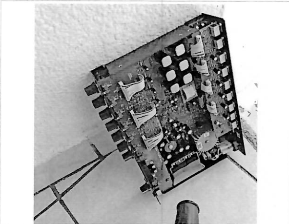
Se retira equipo, y se le quita la tapa, y se aspira el polvo
