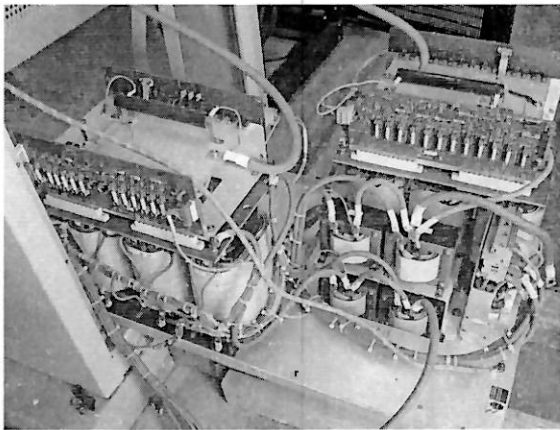
Se retira el carrito de la fuente de poder del transmisor y se ubica la zona de acuerdo a la alarma del transmisor PS2 TAP 1
