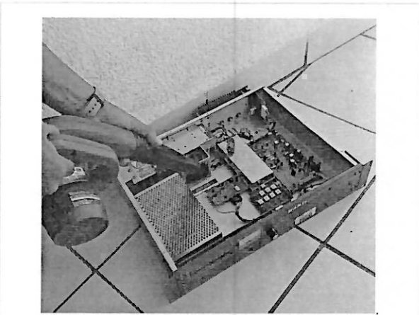
Se extrae el equipo del rack, se destapa y se elimina el polvo de los componentes, principalmente del ventilador de enfriamiento
