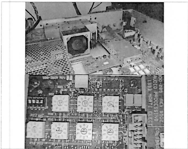
Se pone en operación, y se nota que se elimina el ruido del ventilador, también se verifica la correcta configuración de la frecuencia de operación.
