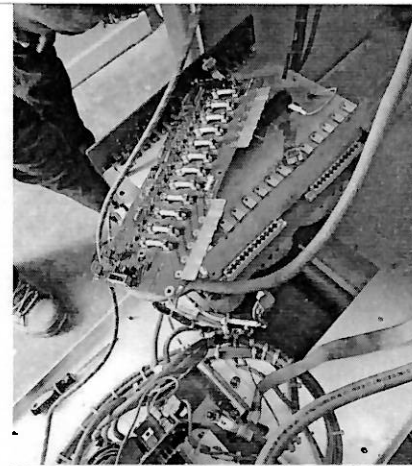
Por una variación fuerte de voltaje (pico alto) se fundió un fusible de la fuente de poder, se detecta el daño y se corrige
