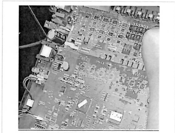
Se limpiaron los potenciómetros con aire comprimido, y se aplica lubricante, se prueban las salidas de audio.
