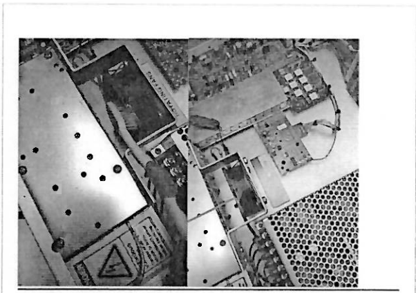
Con aire comprimido y con un cepillo se extrae el polvo del ventilador, y se aplica lubricante especial.
